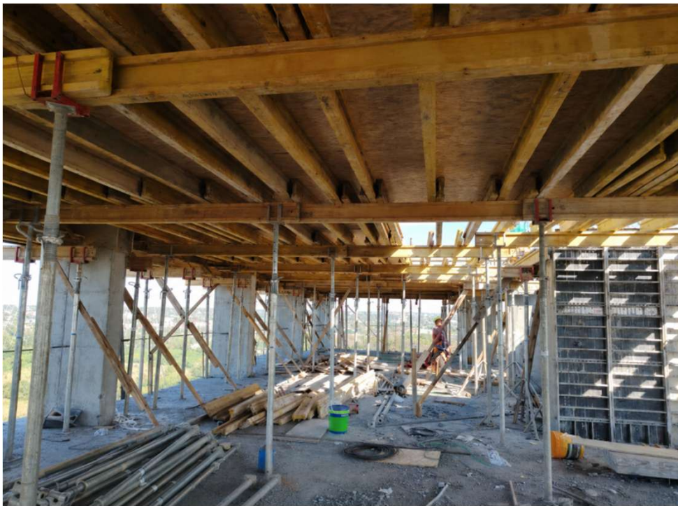
Trabajos de encofrado y armadura de losa
